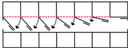
Stallplan mit völlig wegdrehbaren Vorderwänden
